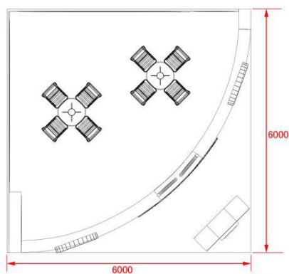
设计方案平面图（范本）
