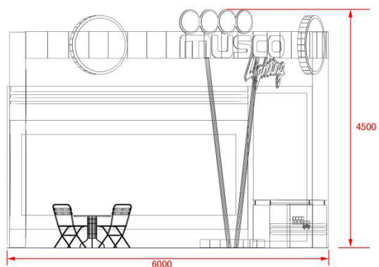
设计方案正立面图（范本）
